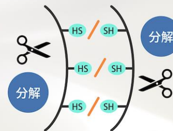
毛の内部での化学反応
